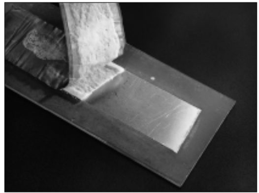
将金属样品浸没10年。请注意胶粘剂粘结层下面的铝材澄亮如新。
